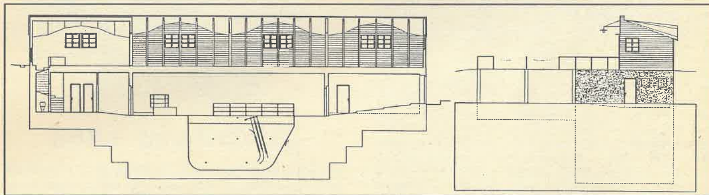
Z řezu budovou je patrné, že ve spodní, z poloviny pod zem schované, části stavby je čistírna odpadních vod. Horní dřevěná nástavba slouží jako sběrna druhotných surovin.
