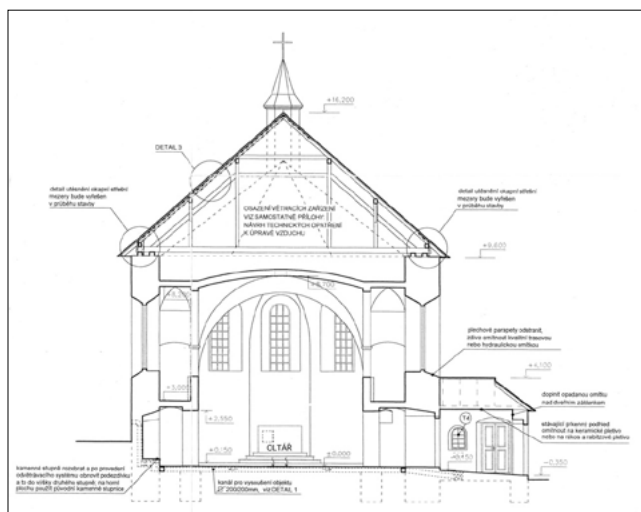
Příčný řez starý kostel, 2004.
