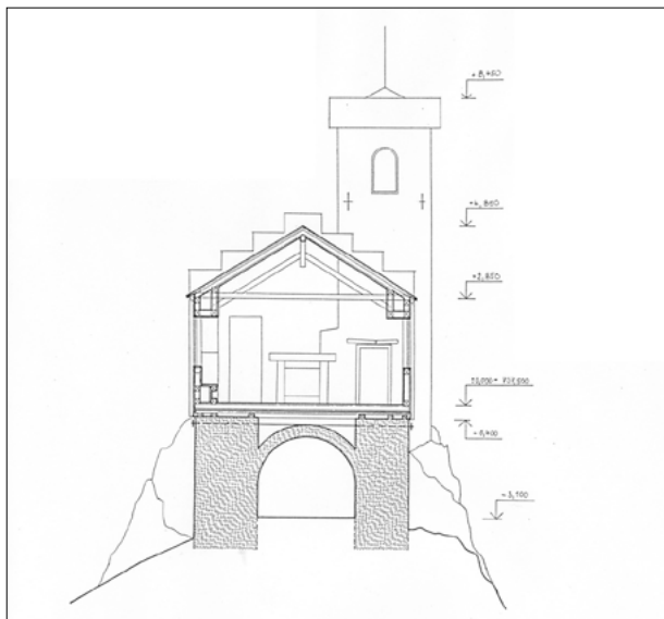
Svislý řez Aichelburg, 1997.
