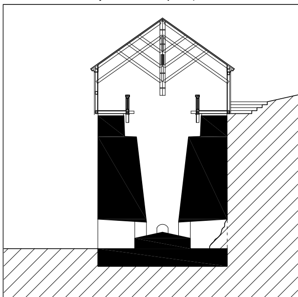
Svislý řez Muzeum Vápenka, 2007.
